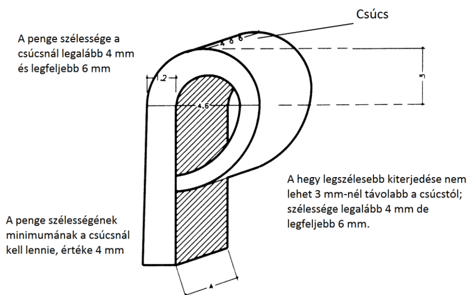
12. ábra Kárd: a kard méretei és hajlékonysága
