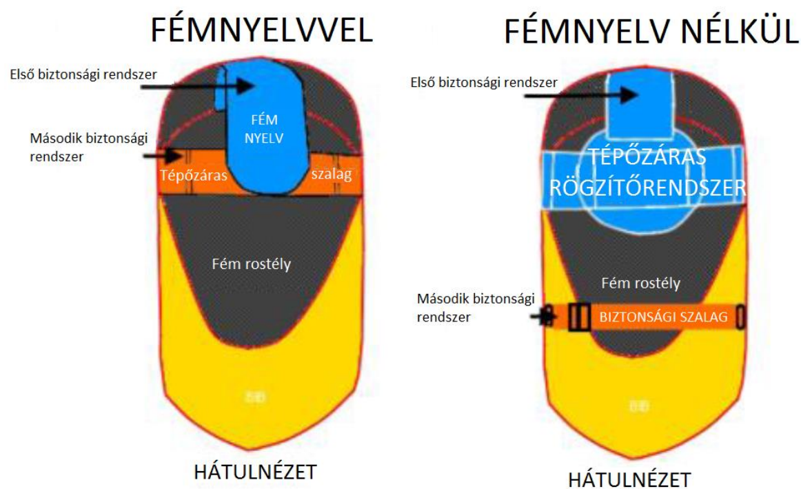
13. ábra: Biztonsági eszközök a fejtéten
